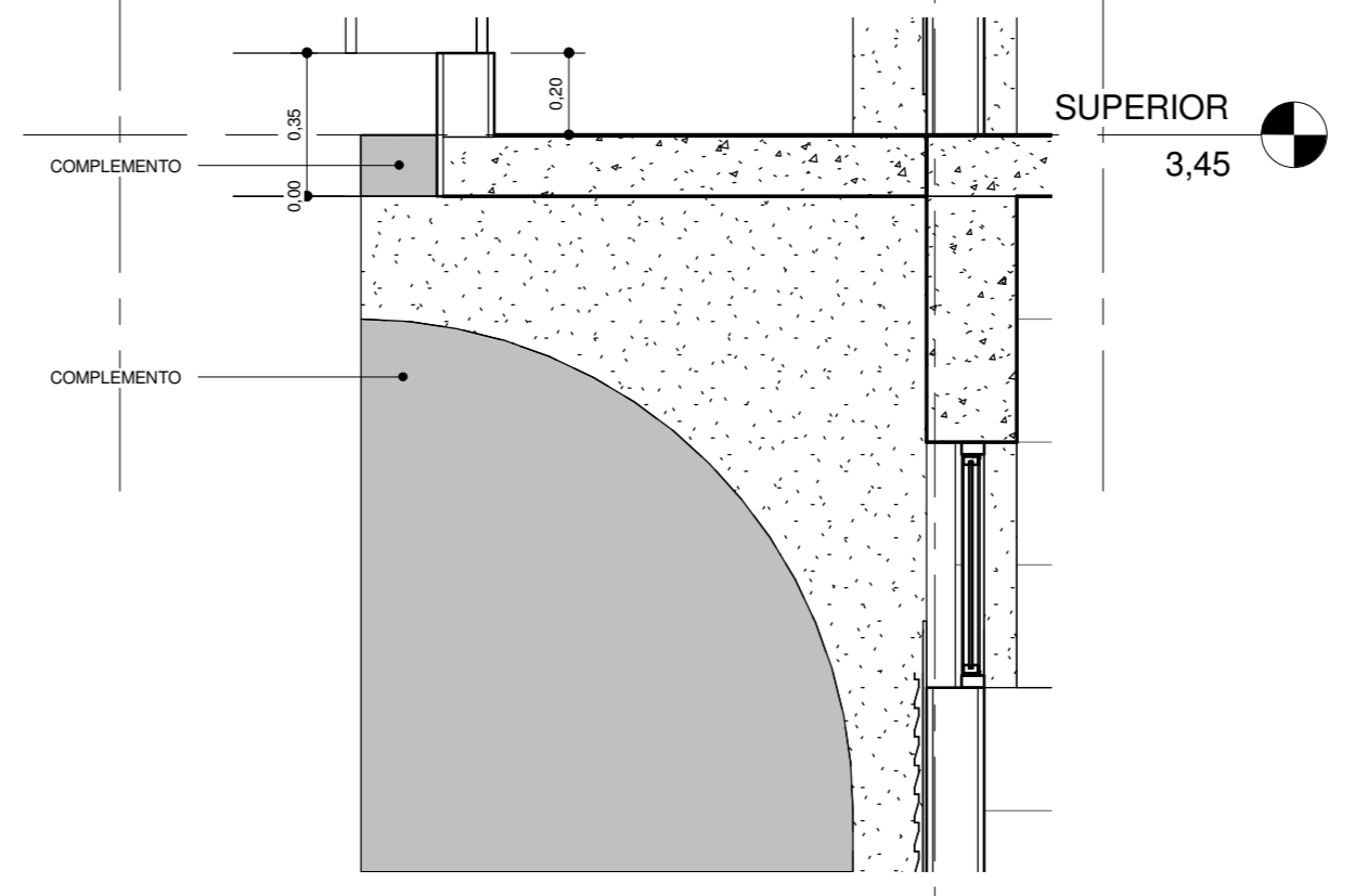
2 Det. Coluna Térreo 1:20
