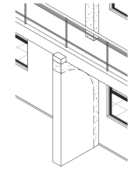
3 Det Coluna Térreo
